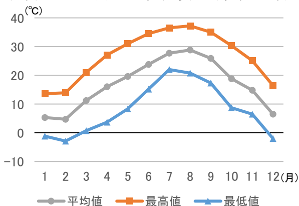
■図表 1-1-5 気温の経月変化(令和4年)
