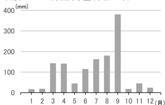
■図表 1-1-3 月別降水量(令和4年)
