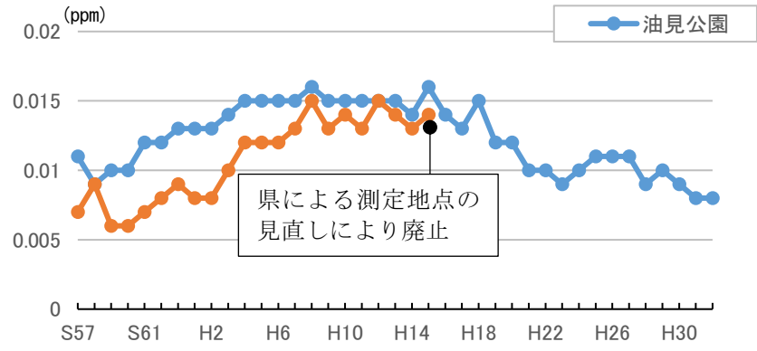
■図表3-1-5 二酸化窒素の経年変化(年平均値)
