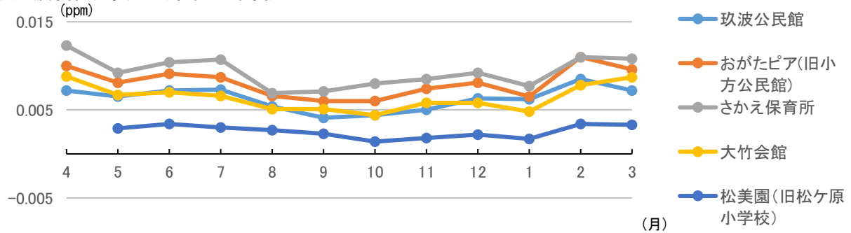
地点別濃度経月変化 (令和2年度)
