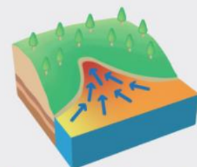
地形による津波の増幅の例
