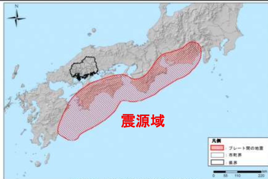
図1.4.1-1 想定地震位置図（南海トラフ巨大地震）
