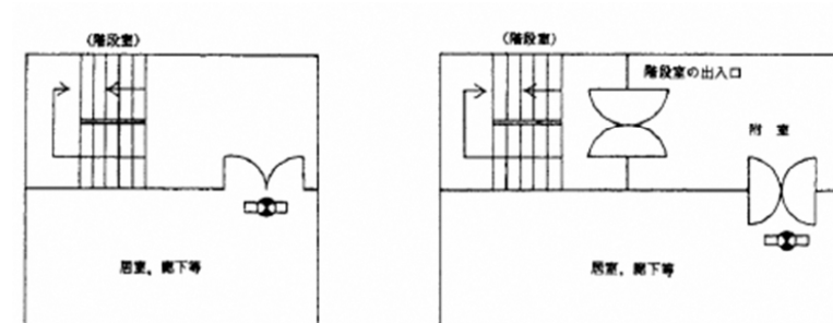
図16-9 避難口誘導灯の設置例
