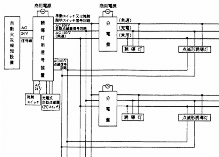
図16-23 機器結線図
