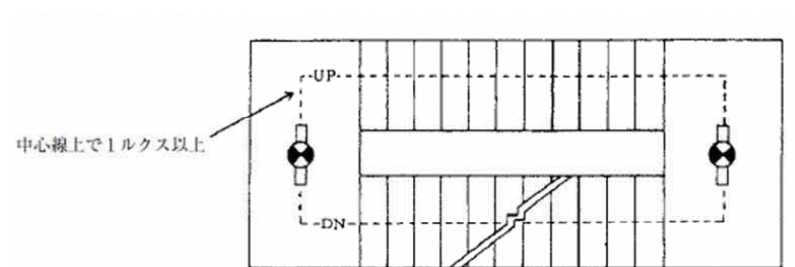
図16-20 階段通路誘導灯の設置例
