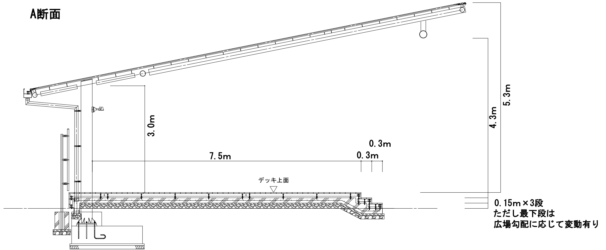
大竹駅西口交流広場ステージ 断面図
