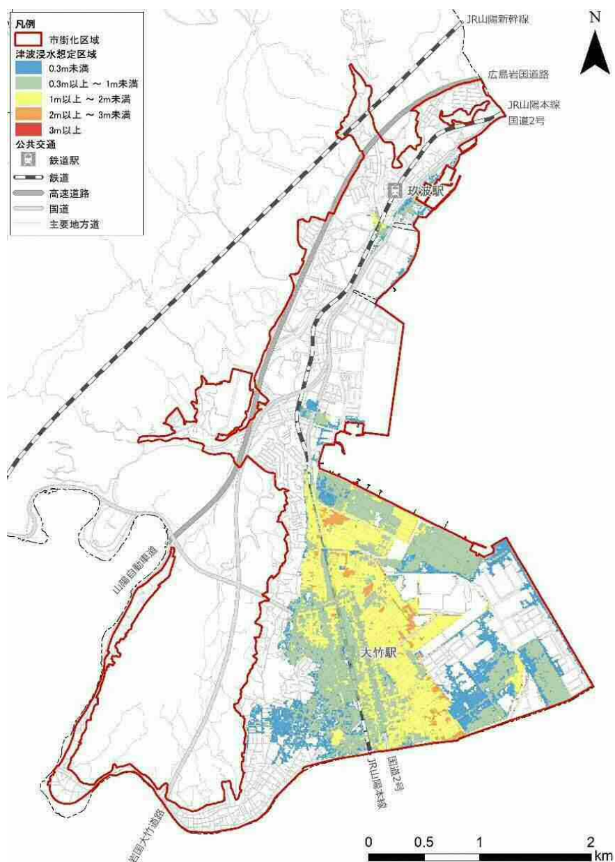
図 8-14 津波浸水深
