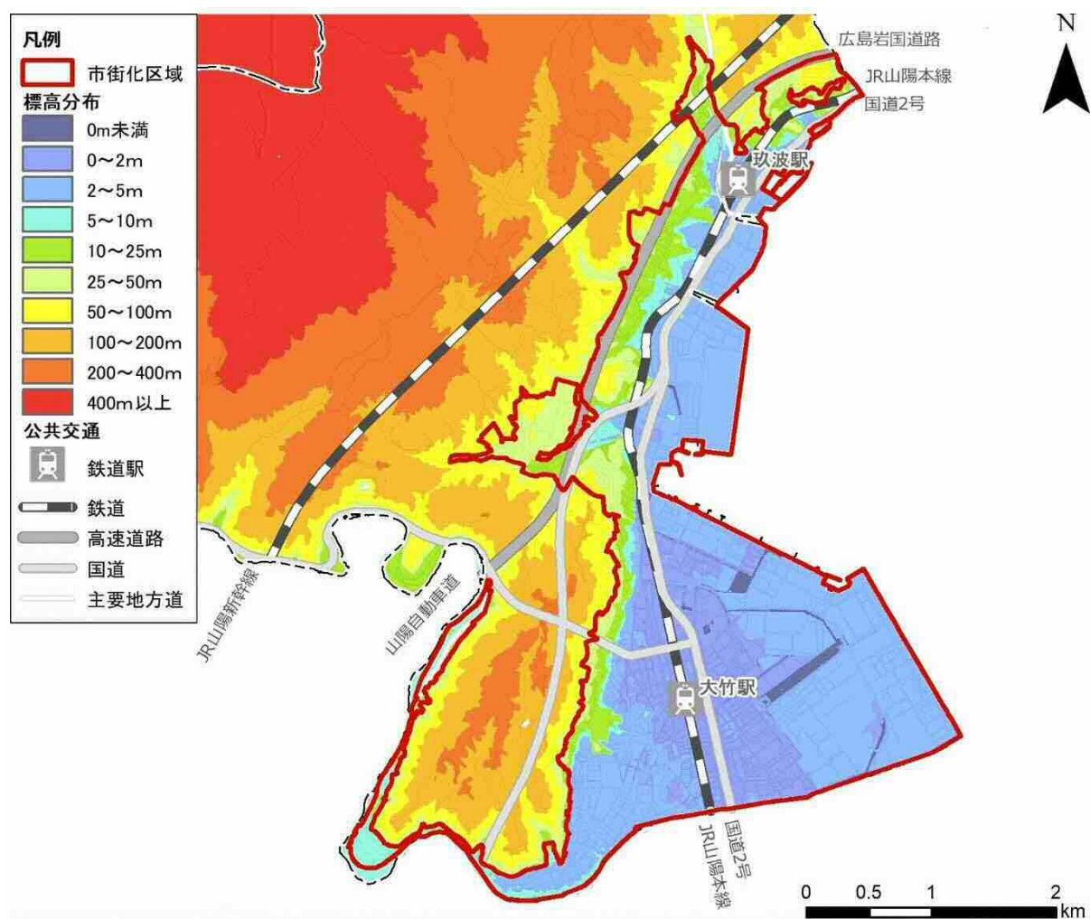
図 8-3 標高分布
