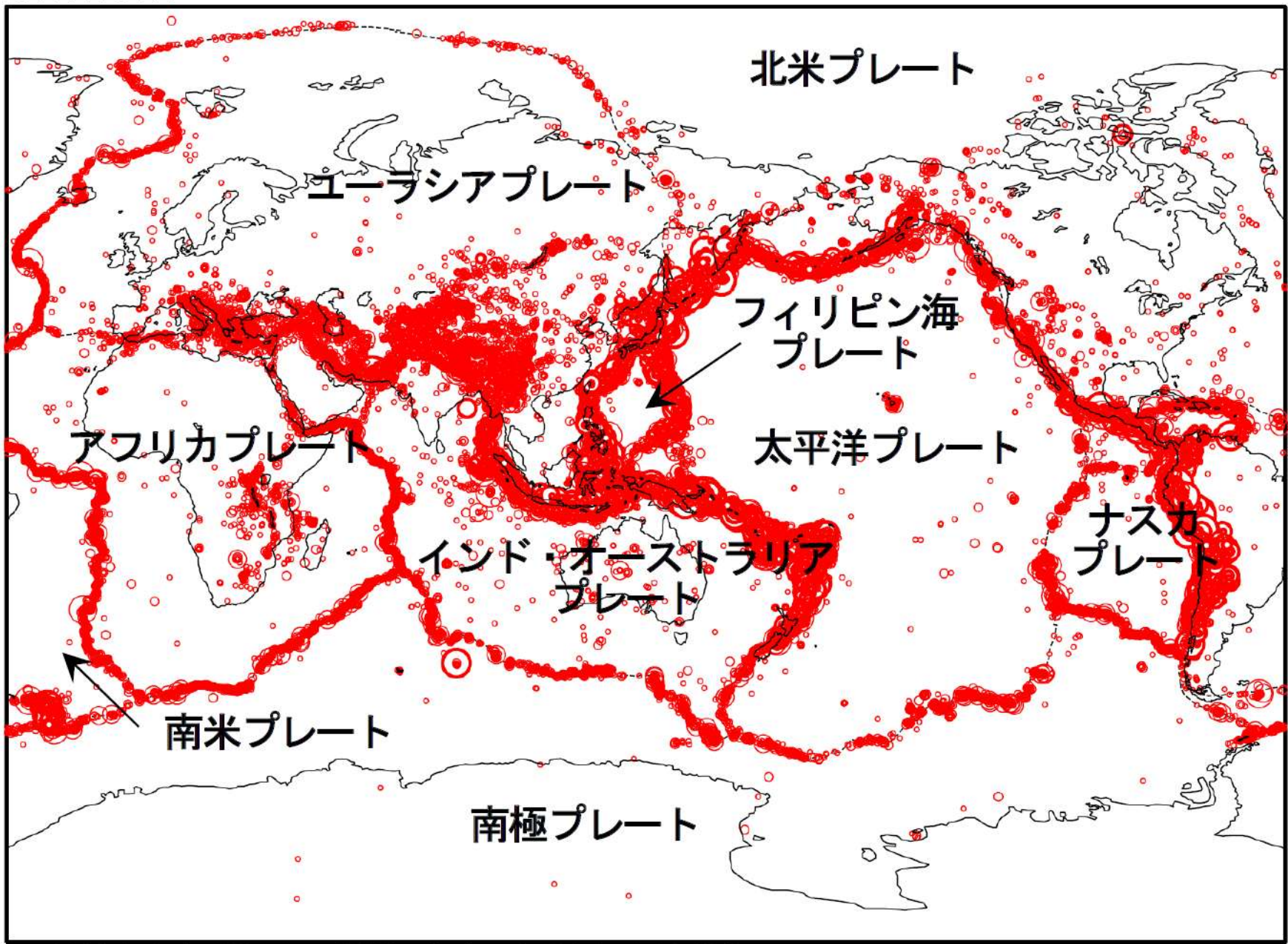
※2011年から2020年の期間に発生した地震の震央分布。 点線は主要なプレート境界。震源データは、米国地質調査所による。
